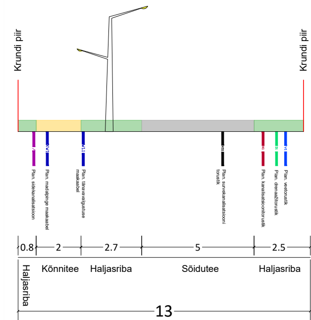
Lõige A - A'
